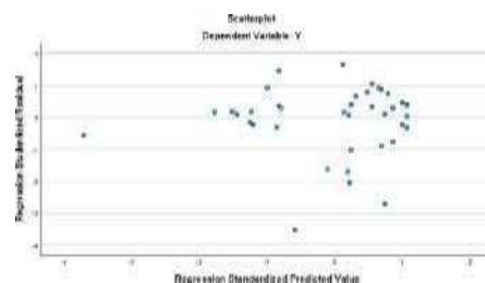
Gambar 2. Uji Heteroskedastisitas
